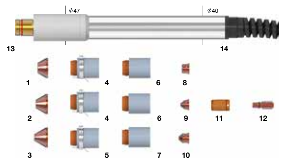
Maschinenhandbrenner XM-160
