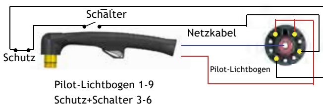
Plasmahandbrenner XT-160
