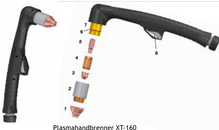
Plasmahandbrenner XT-160
