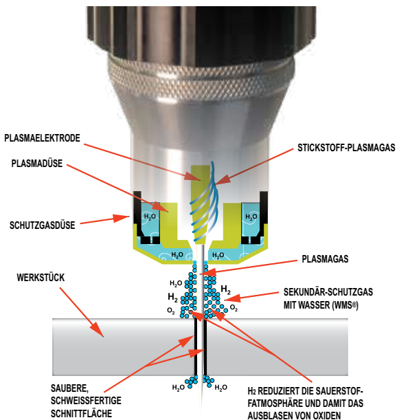
N2 / H2O Plasmaschneiden an Edelstählen
