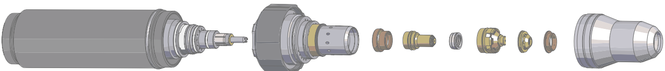
N2 / H2O Plasmaschneiden an Edelstählen
