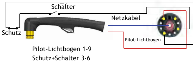
Plasmahandbrenner XT-160
