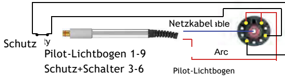
Maschinenhandbrenner XM-160
