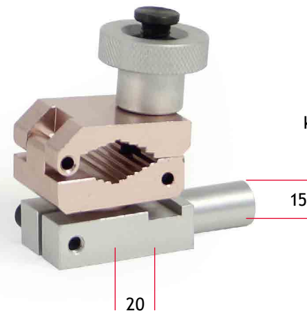
Klemmhalter Typ 6
