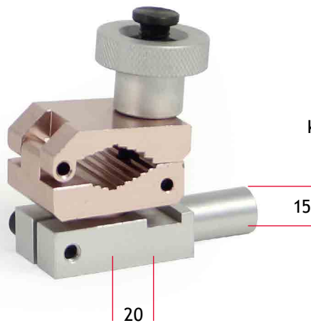
Klemmhalter Typ 6
