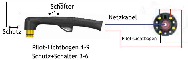
Plasmahandbrenner XT-160
