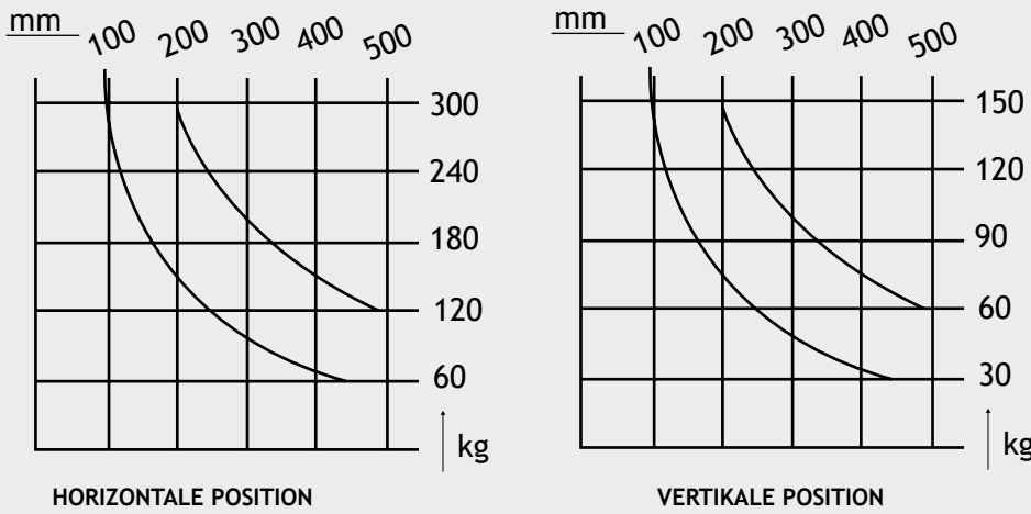
Diagramm: ECO S300
