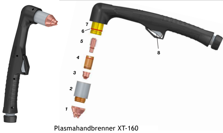
Plasmahandbrenner XT-160
